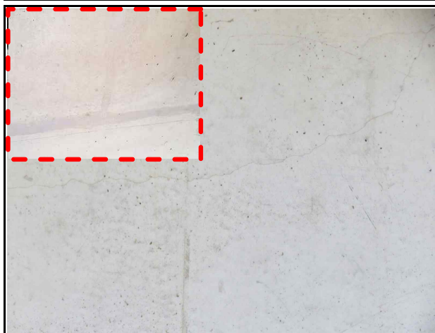
교각 P1(오창방향) 균열(폭 0.1mm)(보수완료)
