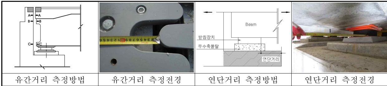
【그림 2.4.11】 부재별 기능상태 측정방법 및 전경
