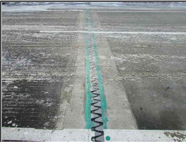
신축이음 상태양호(A2, 오창방향)
