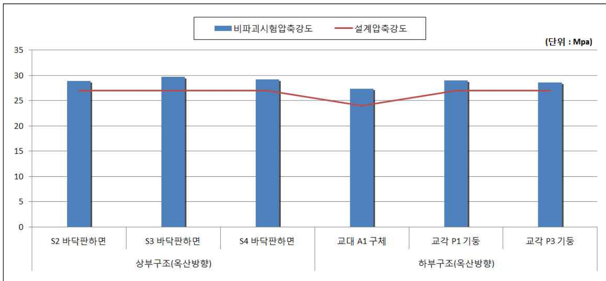
【그림 2.4.6】 콘크리트 강도시험 결과 그래프
