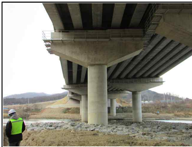
교각 P3(오창방향) 전경
