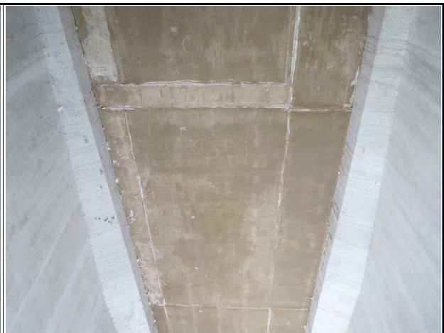
바닥판 하면 상태양호(오창방향)
