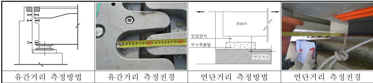
【그림 2.4.5】 부재별 기능상태 측정방법 및 전경
