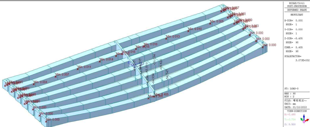
L.C3 하중재하 및 처짐
